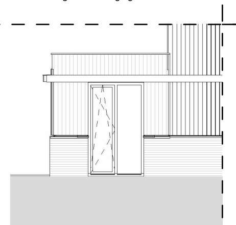
code 10120: uitbouw achtergevel en berging 120cm
