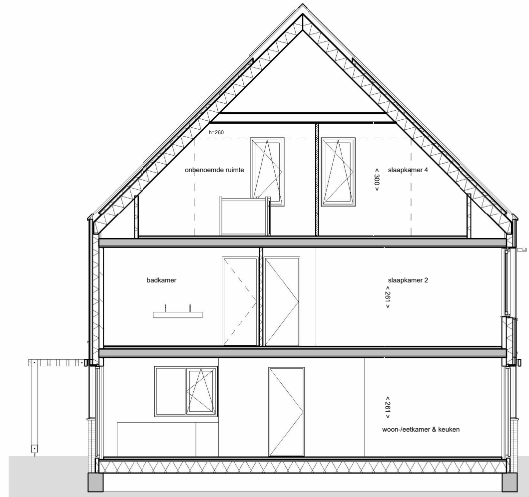
doorsnede B
