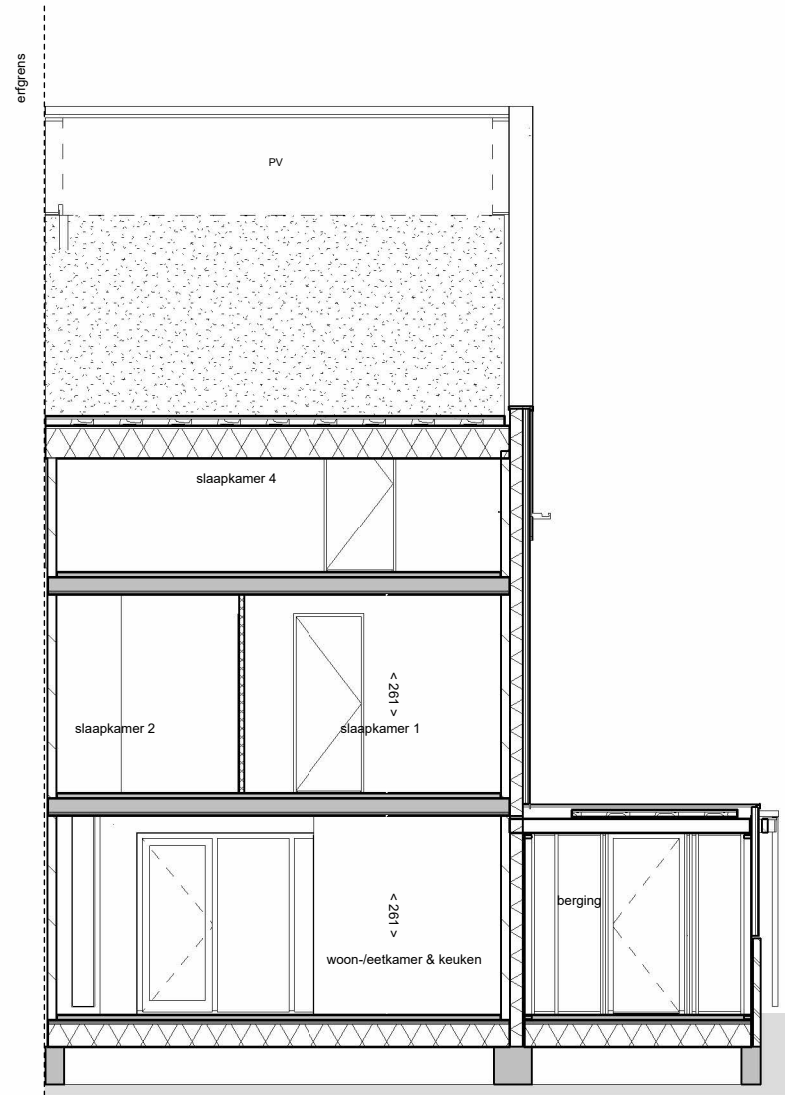
doorsnede A
