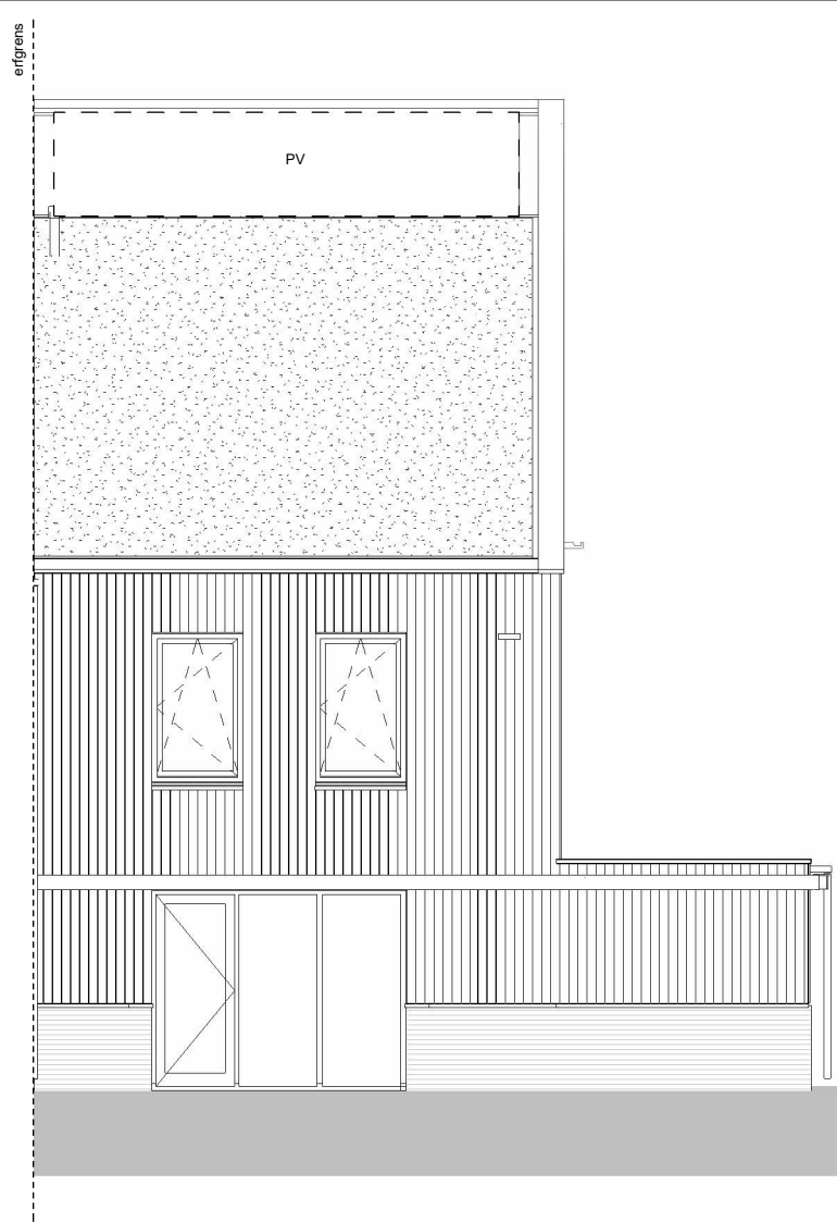
achtergevel
