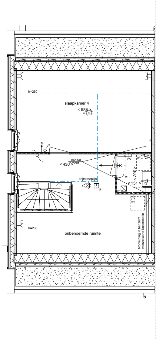
02 tweede verdieping
